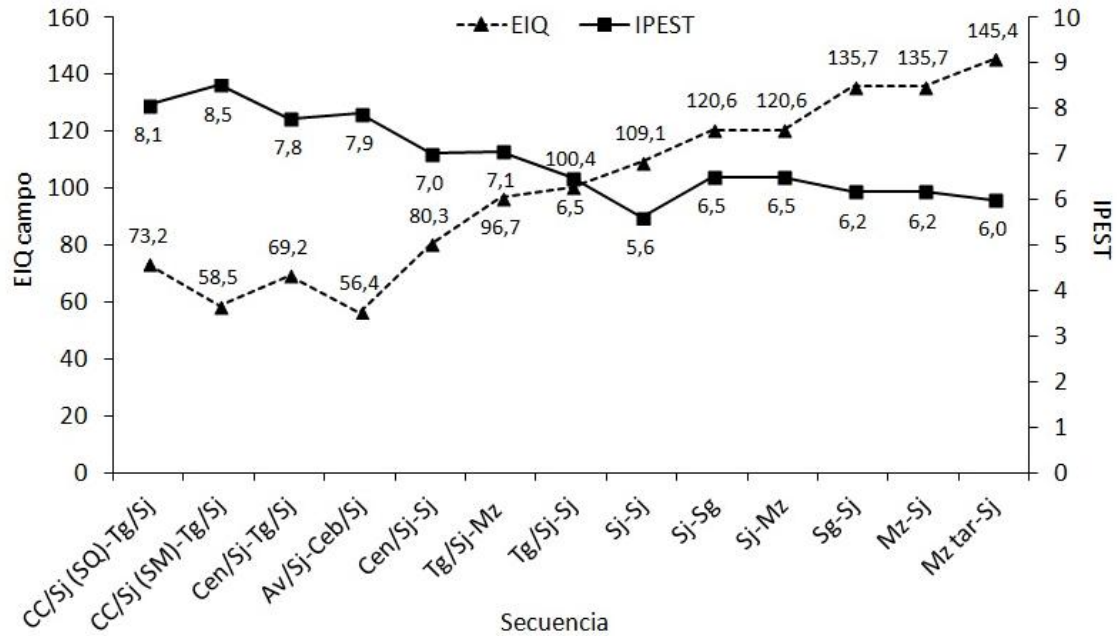
Figura 3. Comparación de índices de coeficiente de impacto ambiental (EIQ) y riesgo ambiental (IPEST) calculados para cada secuencia de cultivos en lotes de producción durante las campañas 2016-17 y 2017-18 en el partido de Pergamino. CC: cultivo de cobertura; SQ: secado químico; SM: secado mecánico; Sj: soja; Cen: centeno; Av: avena; Ceb: cebada; Tg: trigo; Mz: maíz; Sg: sorgo; Mz tar: maíz tardío.
